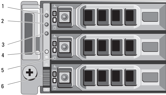
图 2-2. 前面板部件和指示灯 — Dell PowerVault MD3620f
